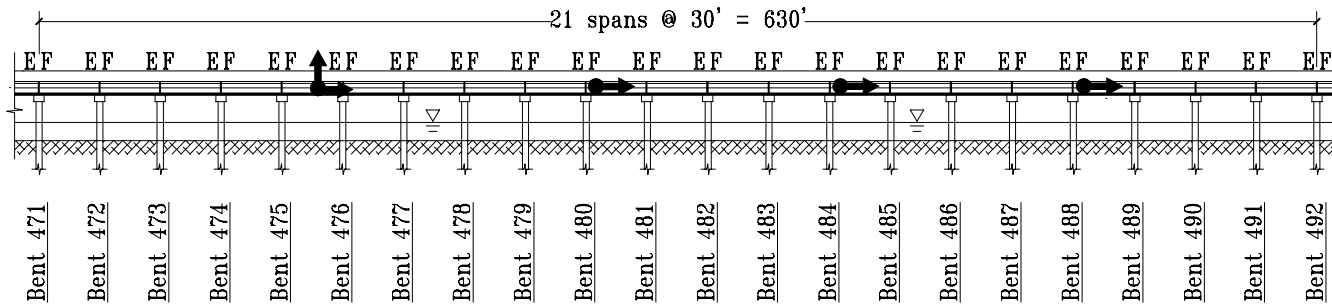
Elevation
