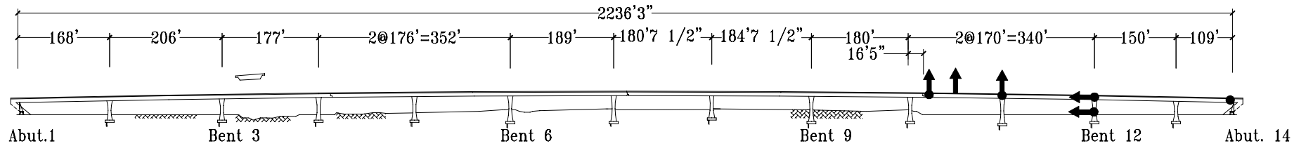
Elevation
