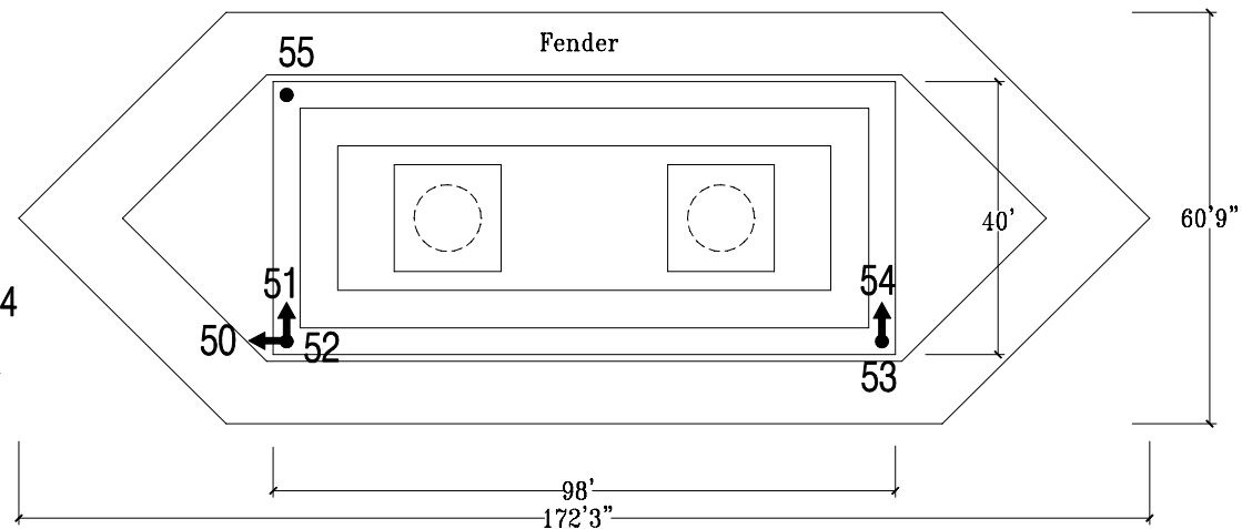
Pile Cap Plan
