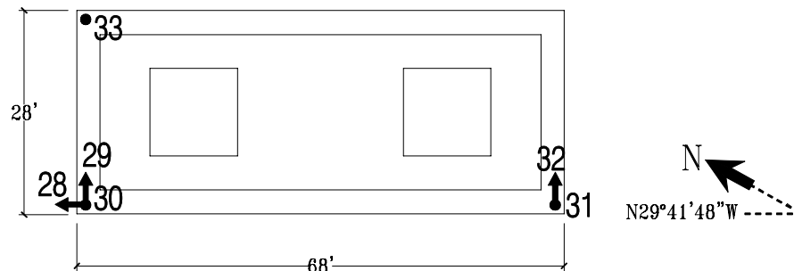
Pile Cap Plan
