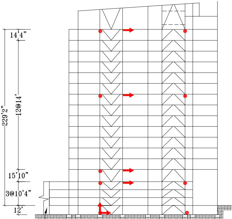
Section A-A'
