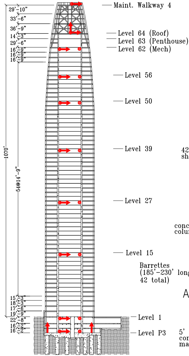
Elevation A-A'
