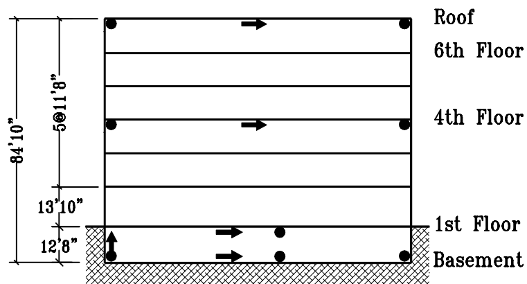
S/N Elevation
