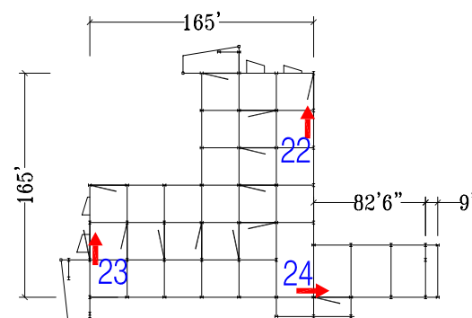
Level 7 (Roof) Plan
