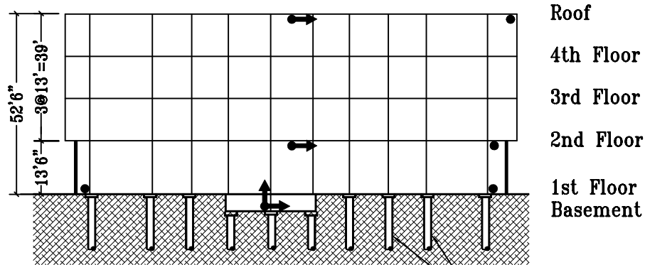
S/N Elevation
