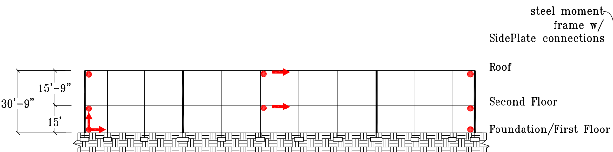
Section A-A'
