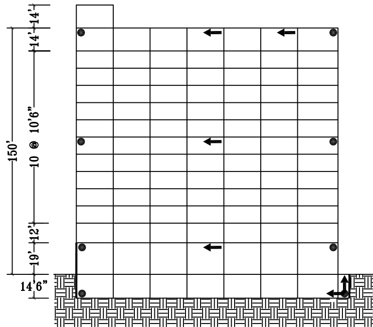
S/N Elevation
