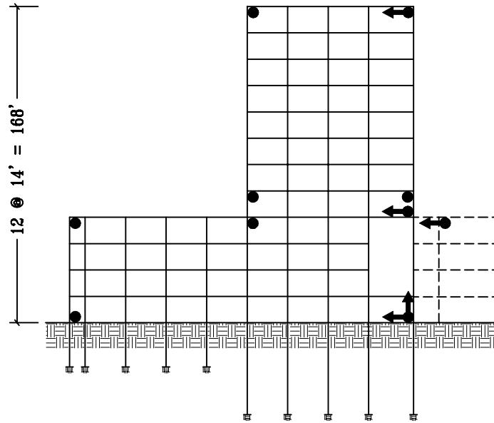
S/N Elevation
