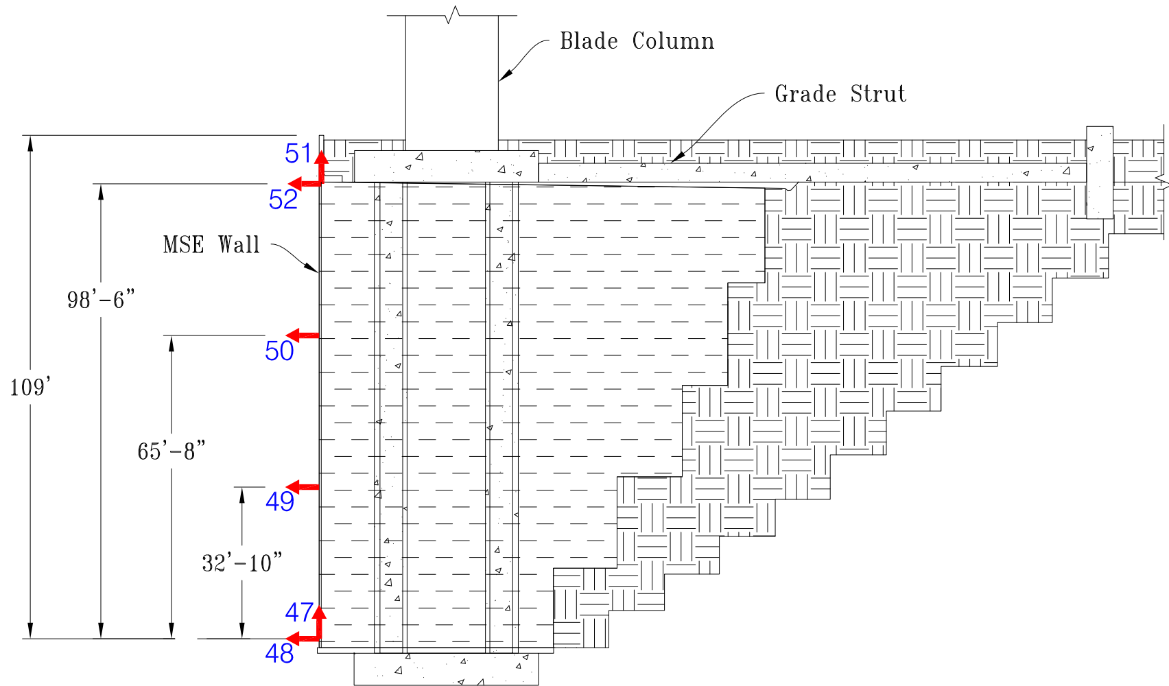
Section A - A' @ MSE Wall
