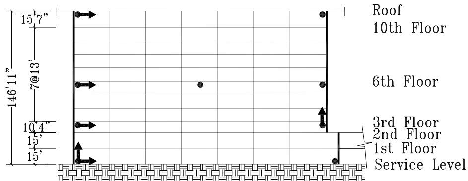
S/N Elevation
