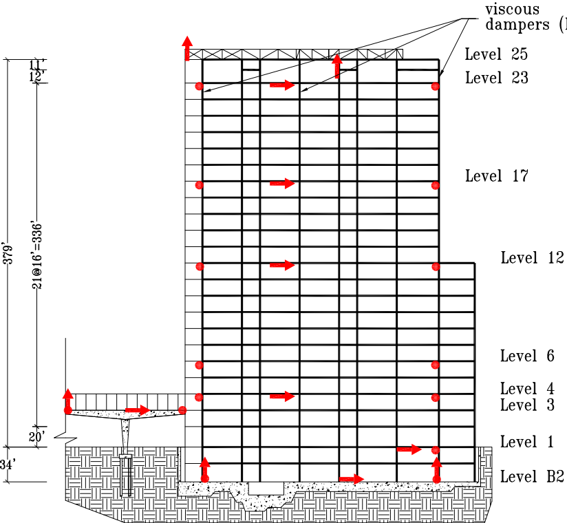
Section A-A'
