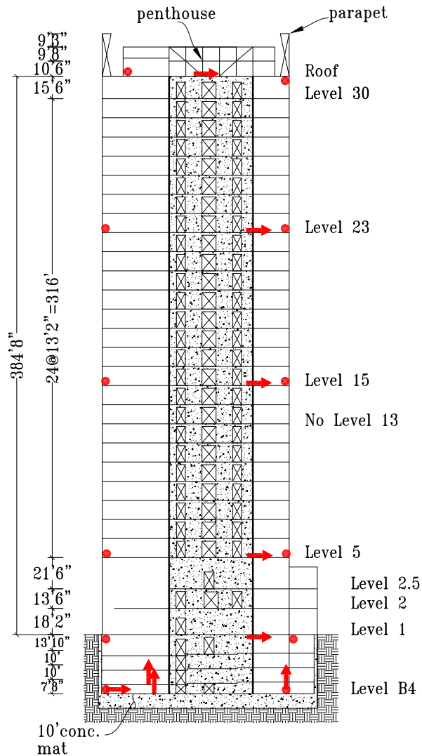
Section A-A'
